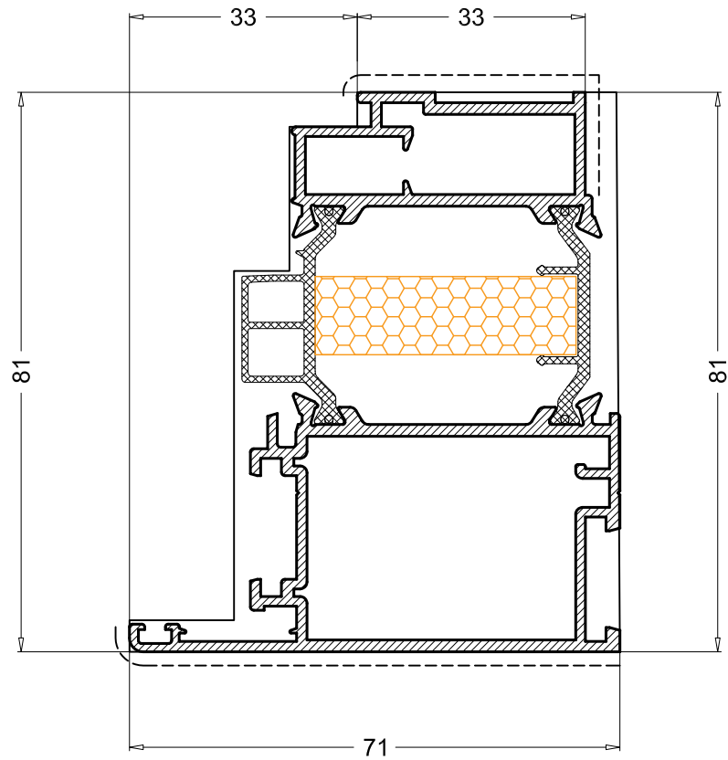
PE85212 1.827 Kg/m
