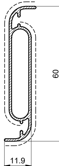
PM 40054 0,413 Kg/m
