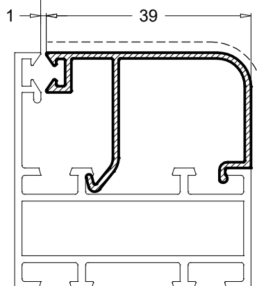
PR58568 0.324 Kg/m
