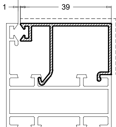
PR58567 0.332 Kg/m
