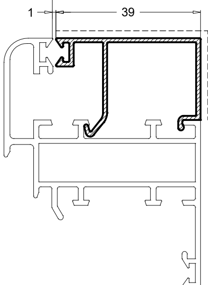
PR58567 0.332 Kg/m
