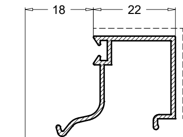
PR58557 0.276 Kg/m
