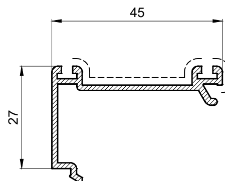
PM 40030 0,413 Kg/m
