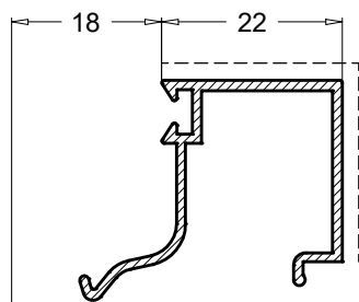
PR58557 0.276 Kg/m
