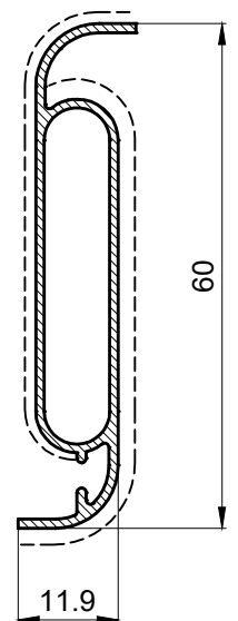
PS 01865 0,379 Kg/m
