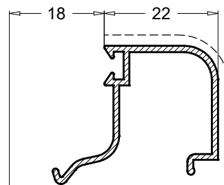
PR58558 0.273 Kg/m
