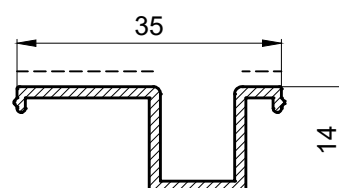
PM 40056 0,254 Kg/m
