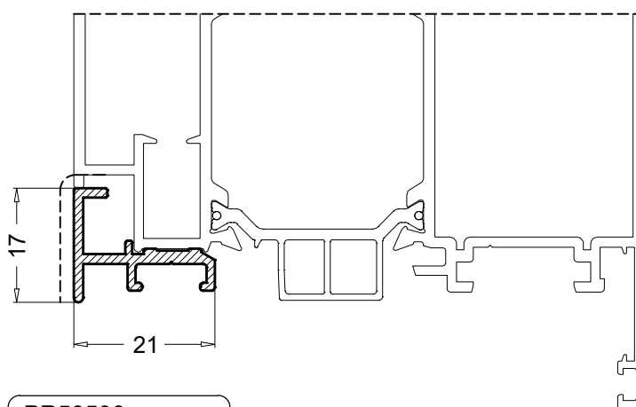
PR58538 0.206 Kg/m
