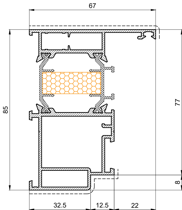
PE85202 1.860 Kg/m
