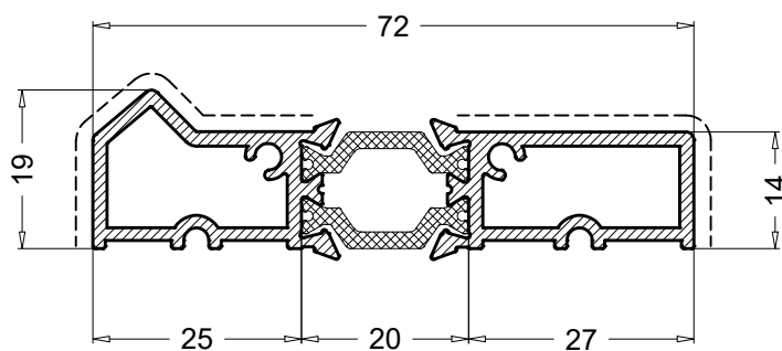
PE85241 0.988 Kg/m
