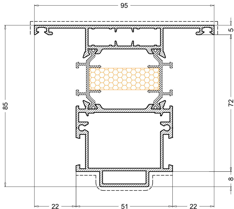
PE85235 2.142 Kg/m
