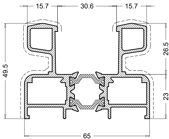
SO65500 1.644 Kg/m
